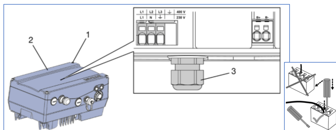
Afbeelding 10: hoofdstroom aansluiting
