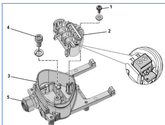
Afbeelding 7: adapterbeugel aansluitblok los
