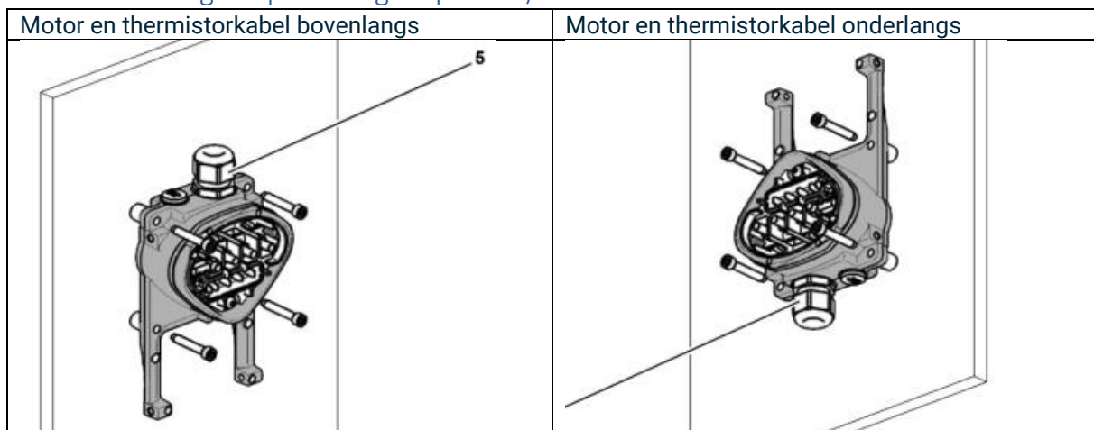
Afbeelding 6: plaatsing adapter beugel
