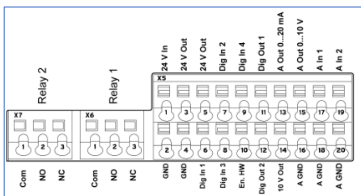
Afbeelding 13: stuurstroomklemmen
