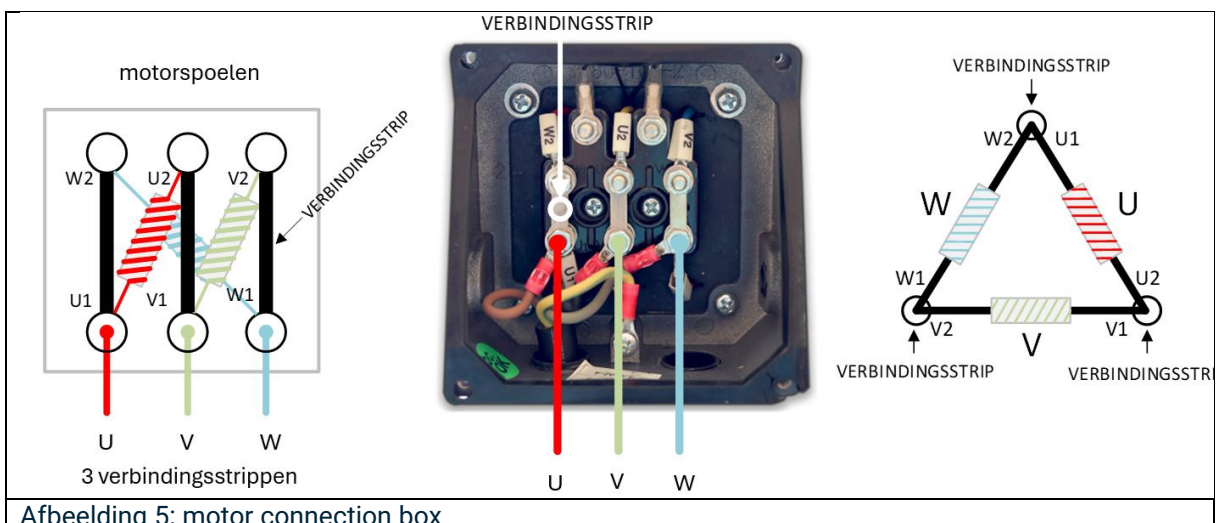
Afbeelding 5: motor connection box
