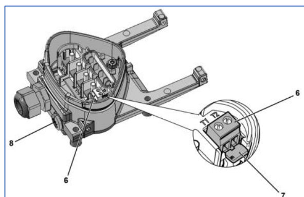
Afbeelding 8: adapterbeugel aansluitblok vast
