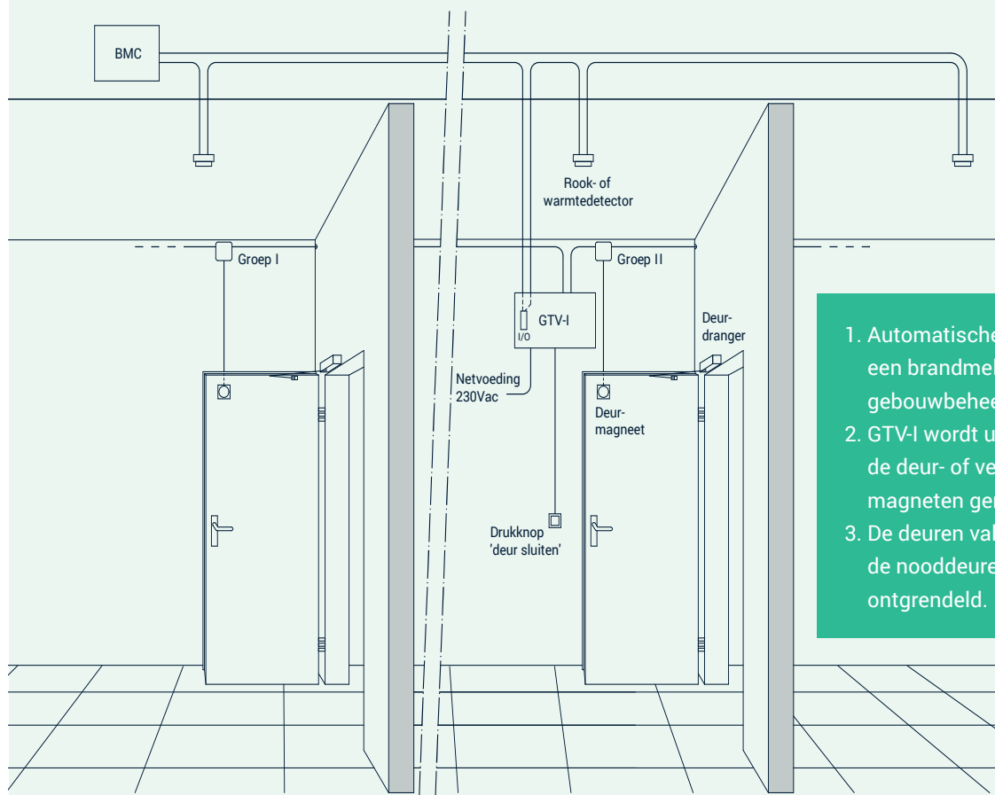
Principe deur ontgrendelsystemen met GTV-voedingen
